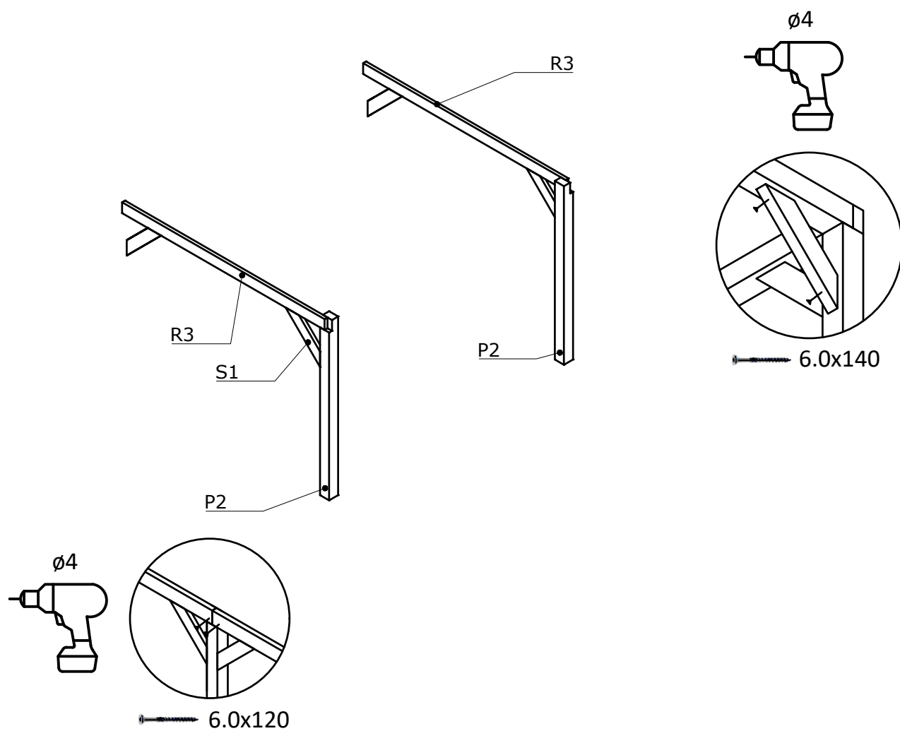
Bovenaanzicht
