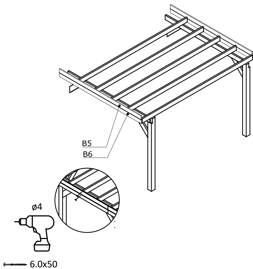
Bovenaanzicht
