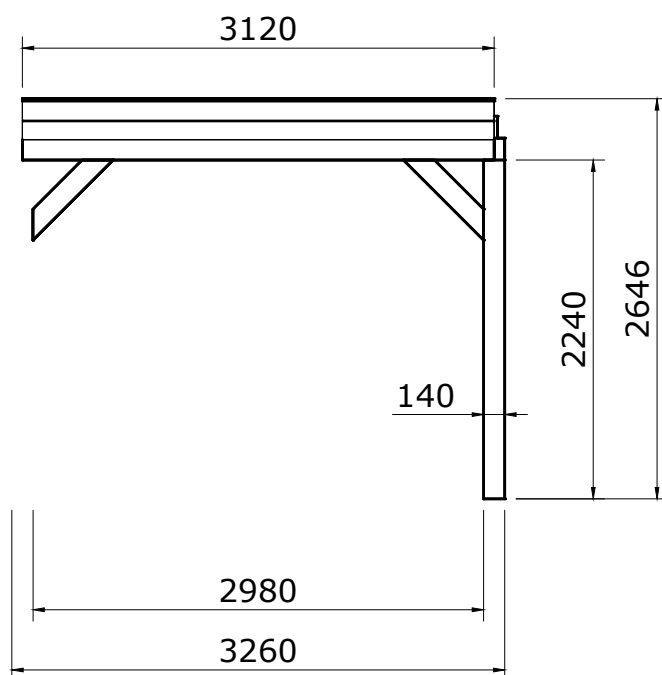
Vooraanzicht
