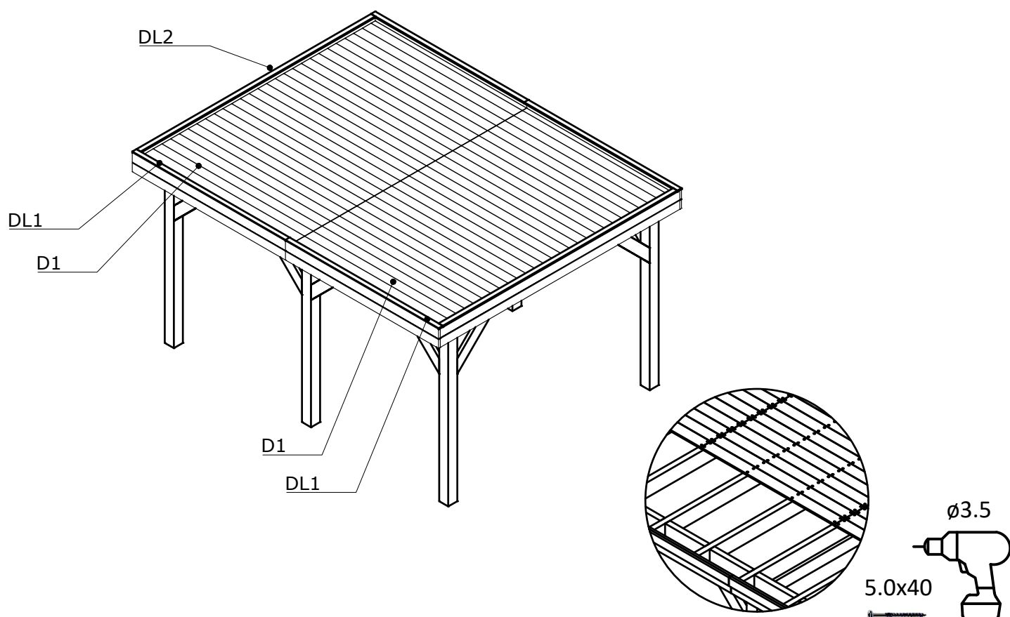
Bovenaanzicht
