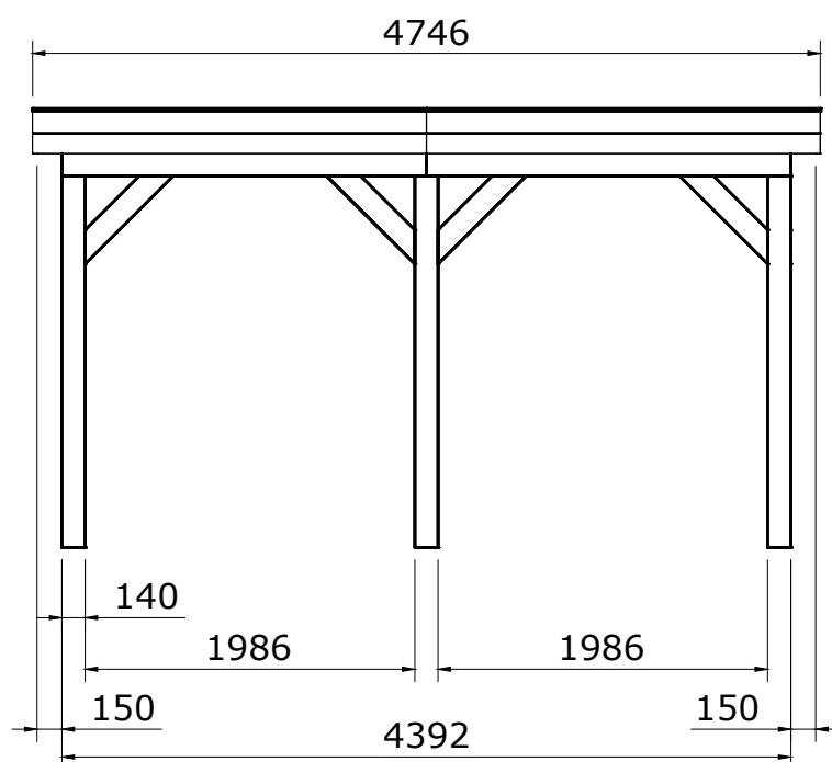
Vooraanzicht
