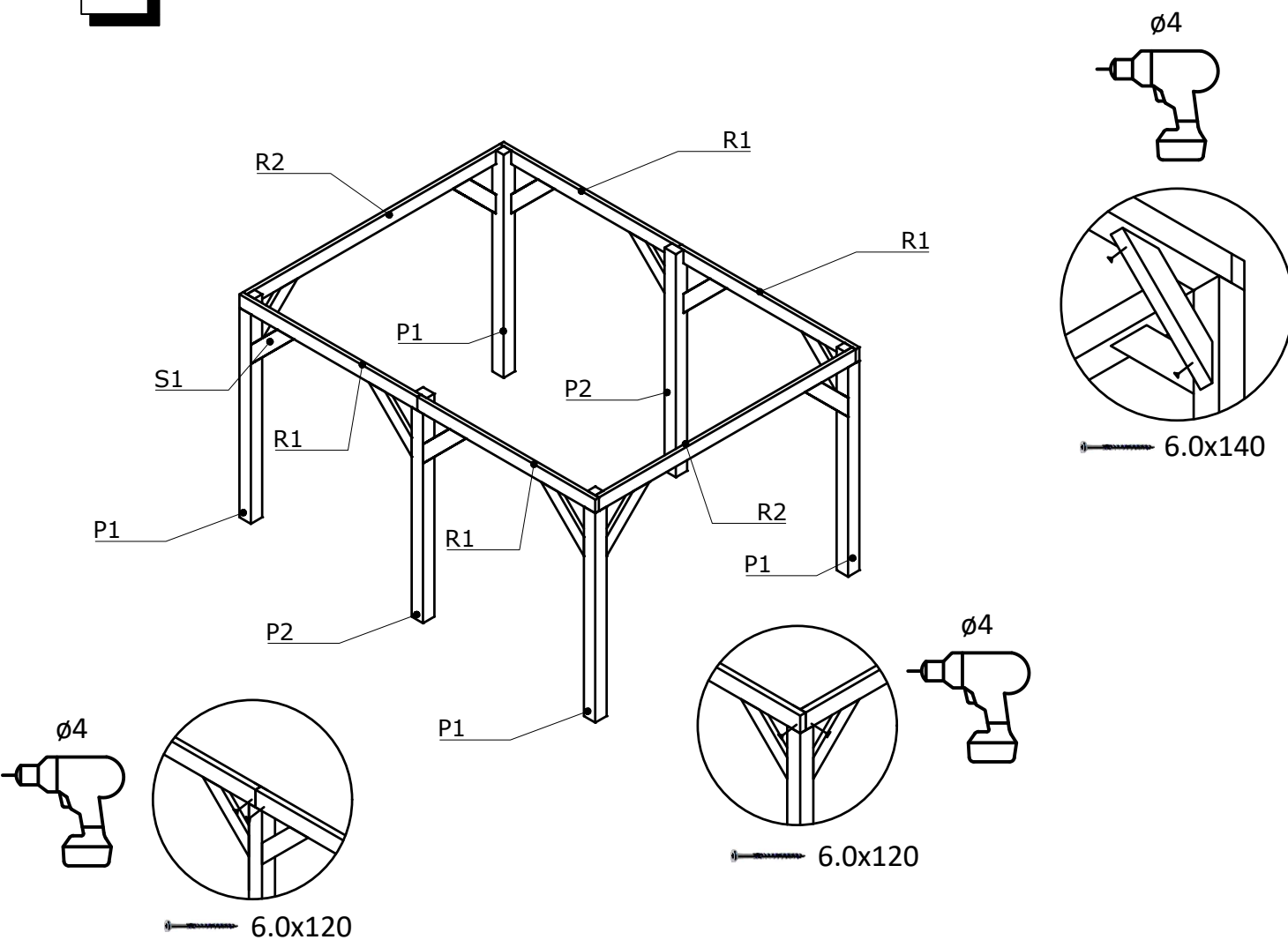
Bovenaanzicht
