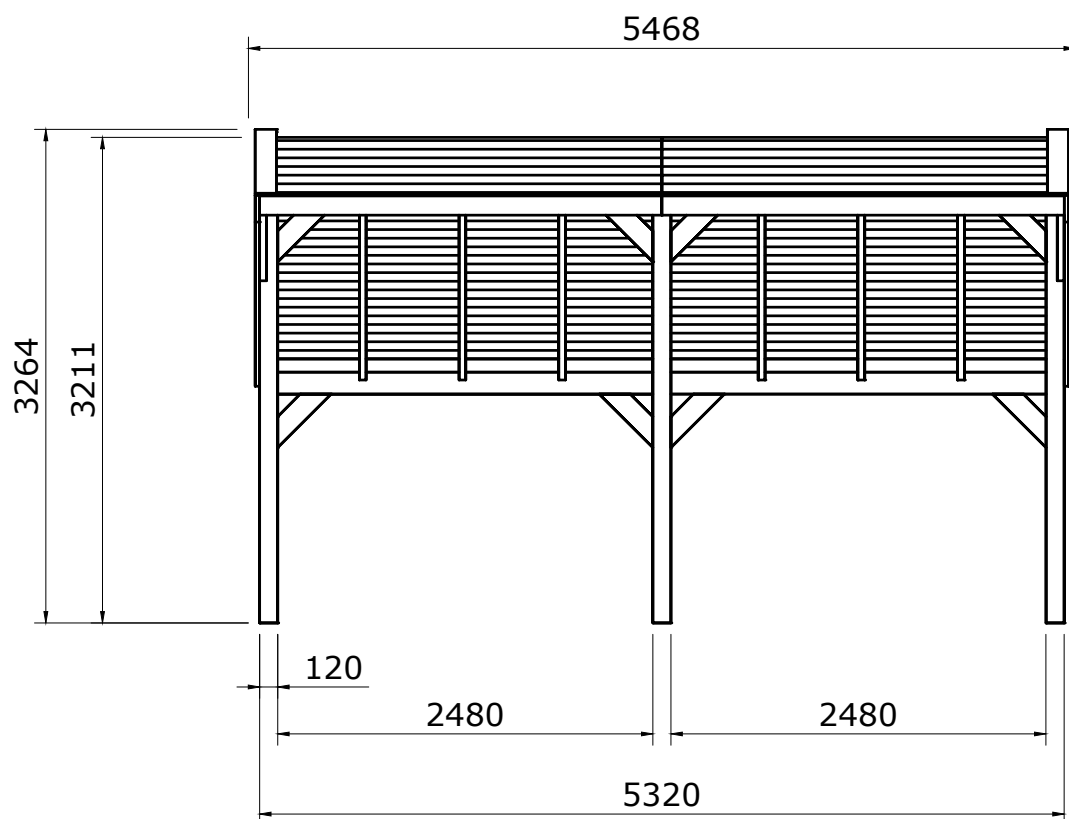
Vooraanzicht
