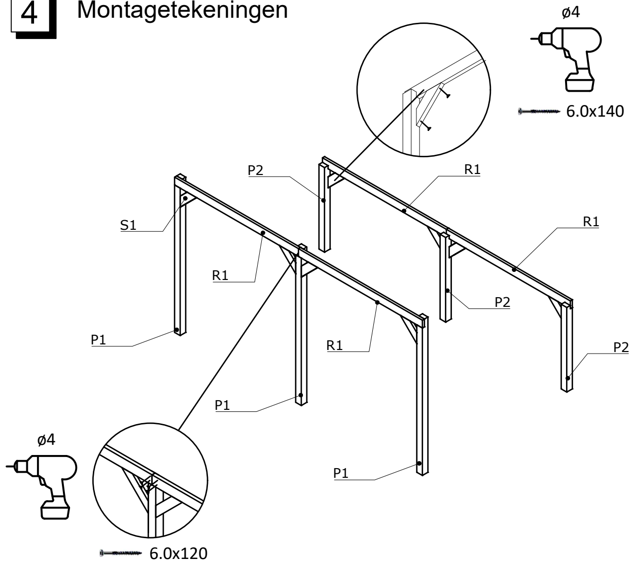
Bovenaanzicht
