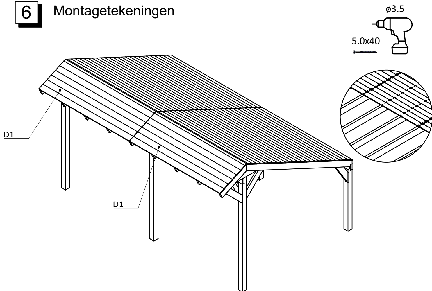
Bovenaanzicht
